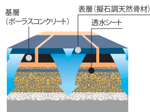
路盤、路床へ浸透
